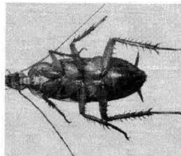
Бегательные конечности
