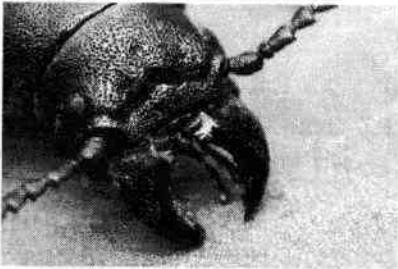
Челюсти
