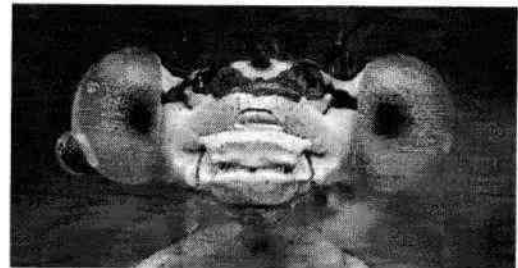
Фасеточные глаза
